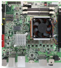
Intel CRB
